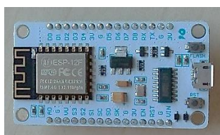
Carte mère : NodeMCU ESP8266
